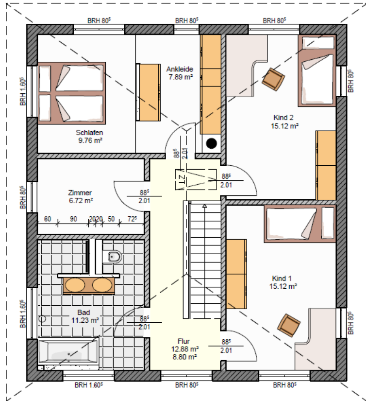
Obergeschoss
