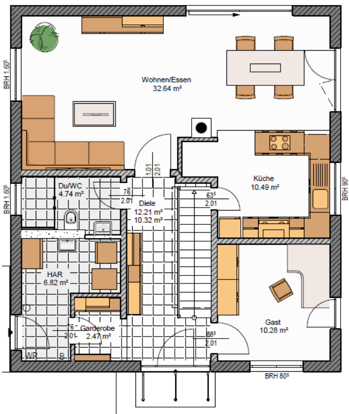
Erdgeschoss
