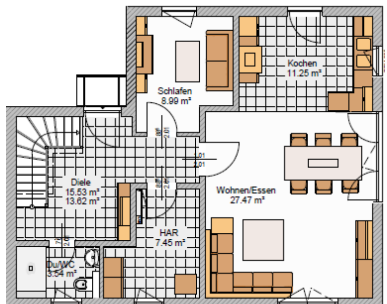
Erdgeschoss
